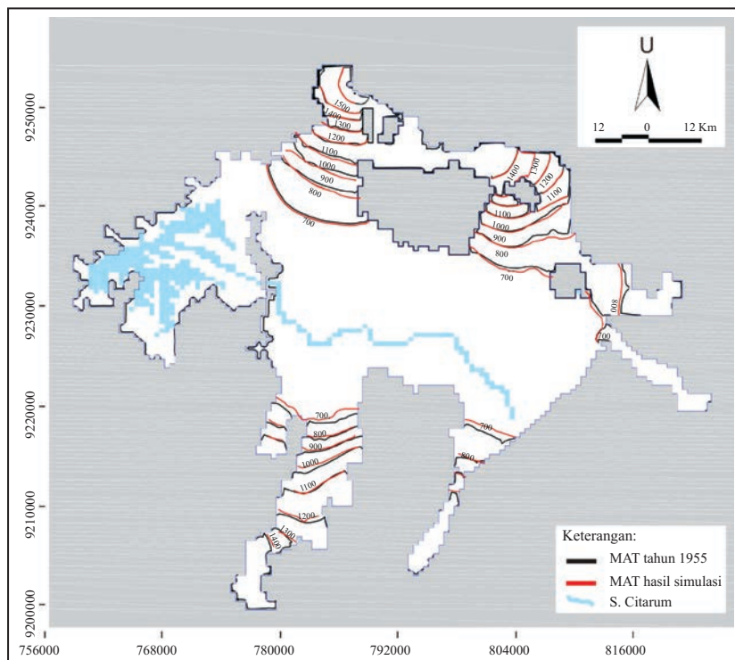
Gambar 6. Kalibrasi hasil simulasi numerik.
