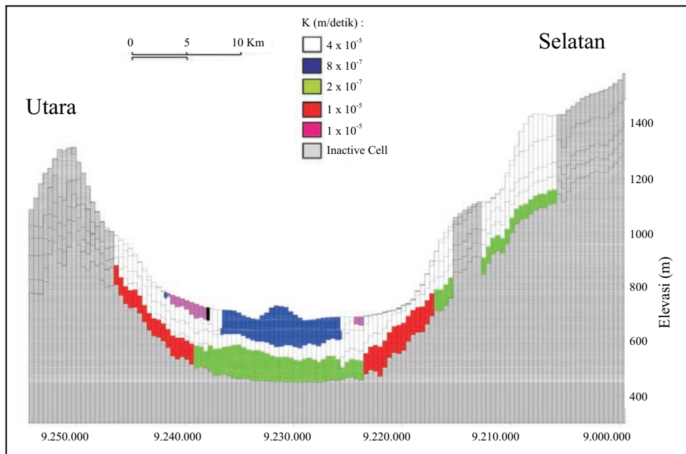
Gambar 5. Contoh penampang hidrogeologi.
