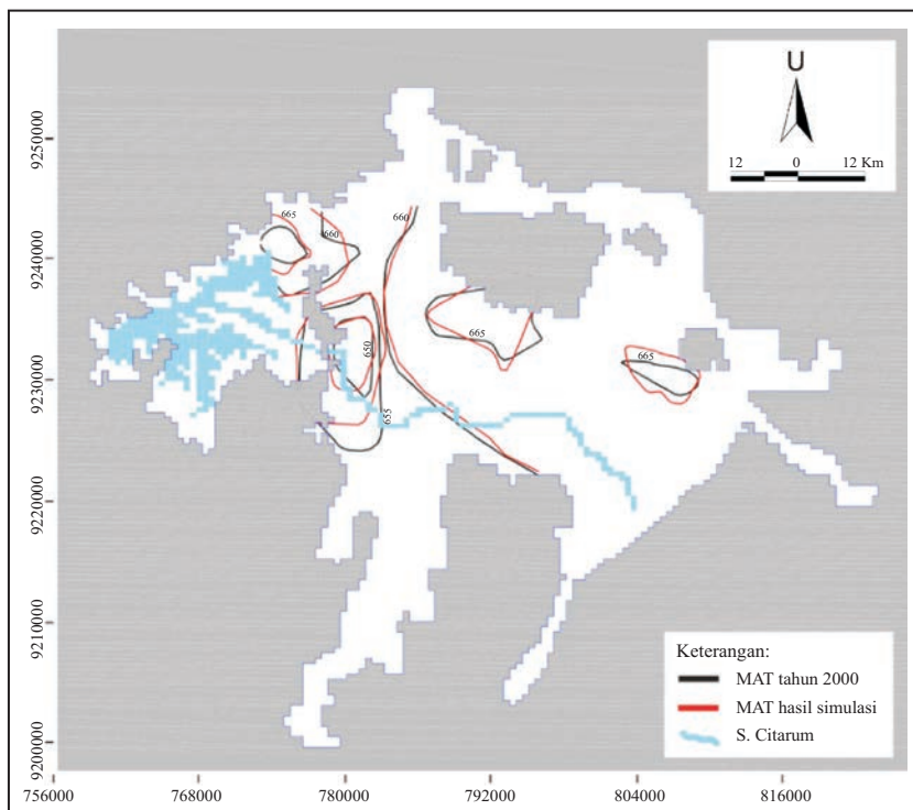
Gambar 7. Verifikasi hasil simulasi numerik.
