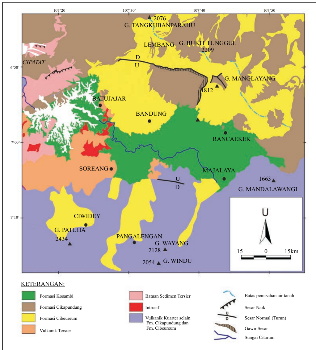
Gambar 2. Peta geologi daerah penelitian, hasil kompilasi dan modifikasi dari Silitonga (1973), Koesoemadinata dan Hartono (1981), Iwaco-Waseco dan PU (1990), Alzwar dr. (1992), Kusmono dr. (1996), dan Sujatmiko (2003).
