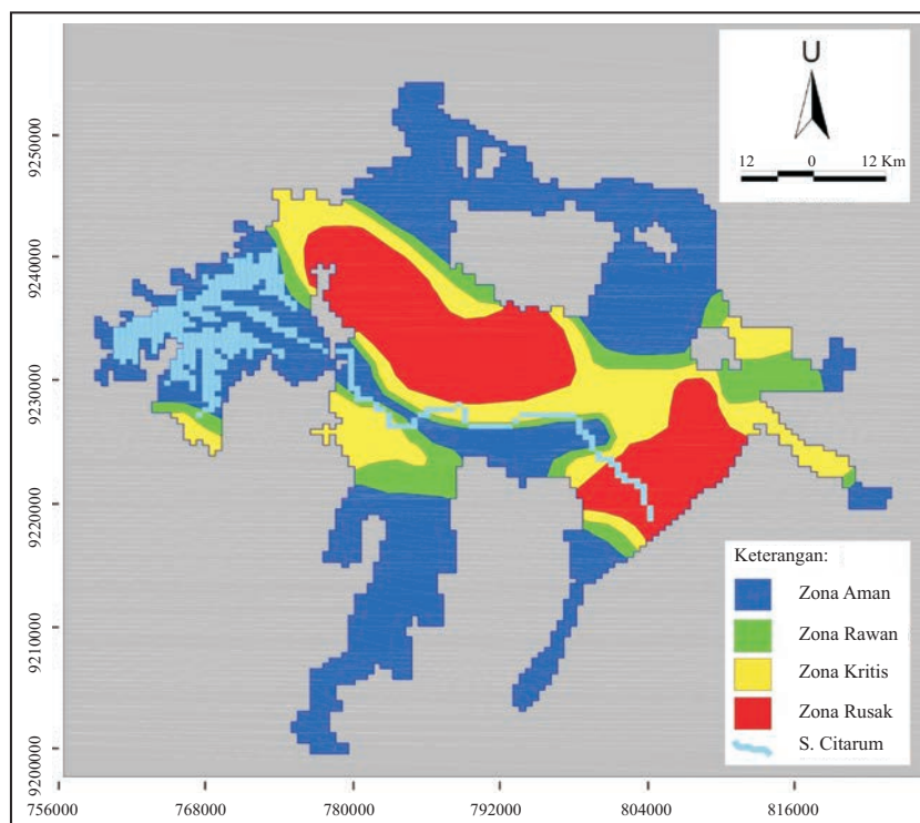
Gambar 9. Zonasi penurunan permukaan air tanah tahun 2013.
