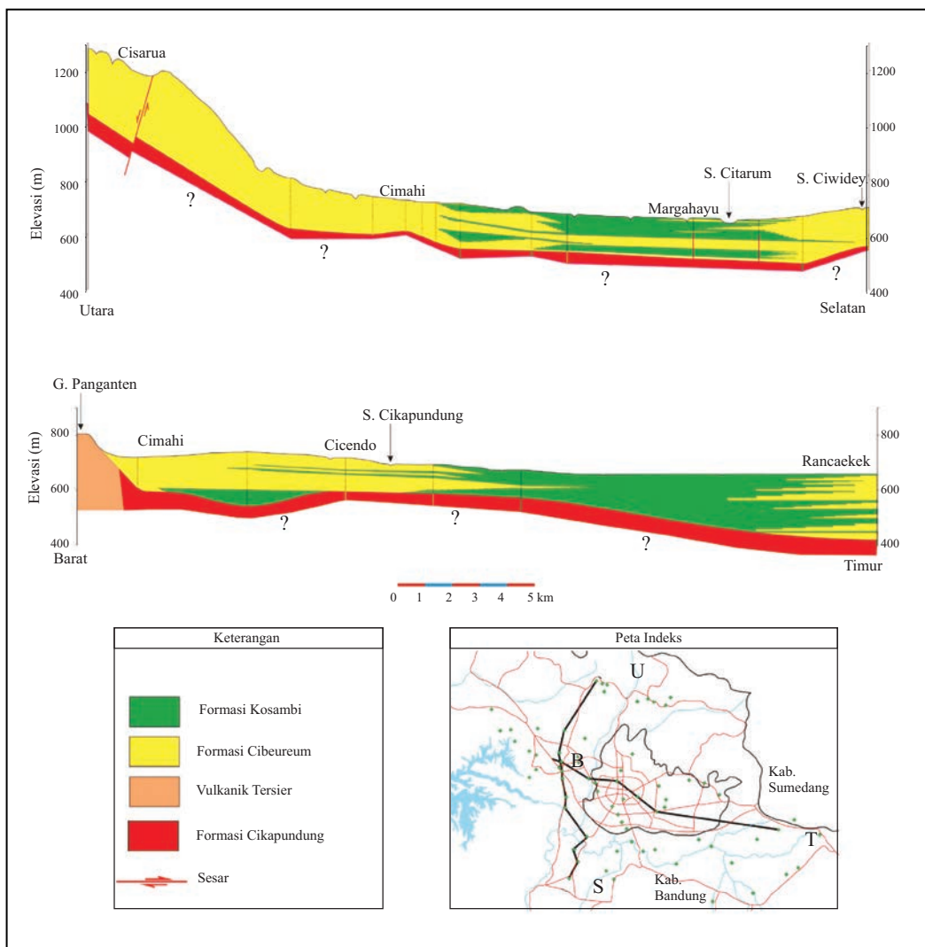
Gambar 3. Penampang geologi daerah penelitian.
