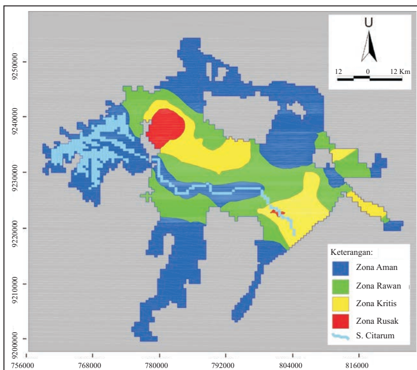
Gambar 10. Zonasi penurunan permukaan air tanah tahun 2000.
