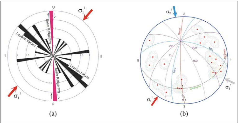
Gambar 9. Diagram mawar yang menunjukkan tegasan utama terbesar ( \sigma_1^I ) pada zaman Tersier berarah U40°T-U230°T. Warna hitam adalah jurus batuan Tersier dan warna merah muda adalah jurus Sesar Kaligarang. Tegasan inilah yang menggerakkan Sesar Kaligarang sebagai sesar menganan (a). Analisis Sesar Kaligarang pada lokasi SMG 06 menghasilkan kedudukan sesar U179°E/83°. Tanda panah warna merah adalah tegasan utama terbesar ( \sigma_1^I ), panah biru adalah tegasan utama menengah ( \sigma_2^I ) dan panah hitam adalah tegasan utama terkecil ( \sigma_3^I ).
