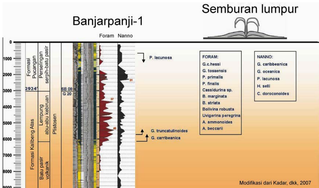
Gambar 6. Biostratigrafi sumur Banjarpanji 1, daerah Porong, Kabupaten Sidoarjo (modifikasi dari Kadar dr., 2007).
