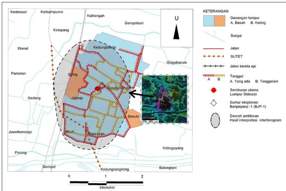
Gambar 8. Hasil analisis interferogram oleh Deguchi drr., 2007.
